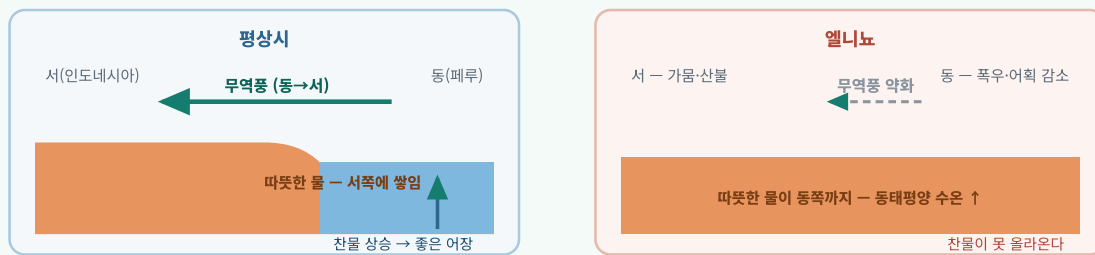
정상시 vs 엘니뇨 — 적도 태평양의 단면
