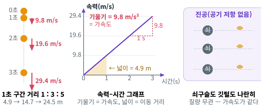
그림 2 | 자유 낙하 — 가속도 약 9.8 \text{ m/s}^2 (매초 9.8 m/s씩), 공기 저항이 없으면 질량과 무관하게 함께 떨어진다
