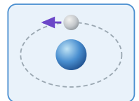
(다) 지구 둘레를 도는 달
