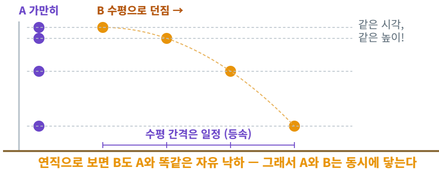
그림 3 | 수평으로 던진 공의 운동 — 수평 등속 + 연직 자유 낙하, 두 운동은 서로 독립이다
