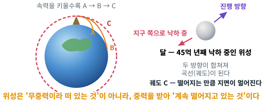
그림 4 | 뉴턴의 사고 실험 — 수평 속력이 충분히 크면 낙하가 궤도가 된다
