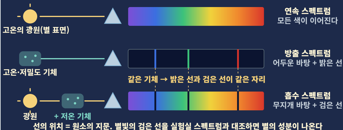
그림 4 | 스펙트럼의 세 종류 — 연속 · 방출 · 흡수. 같은 원소의 방출선과 흡수선은 항상 같은 위치에 나타난다
