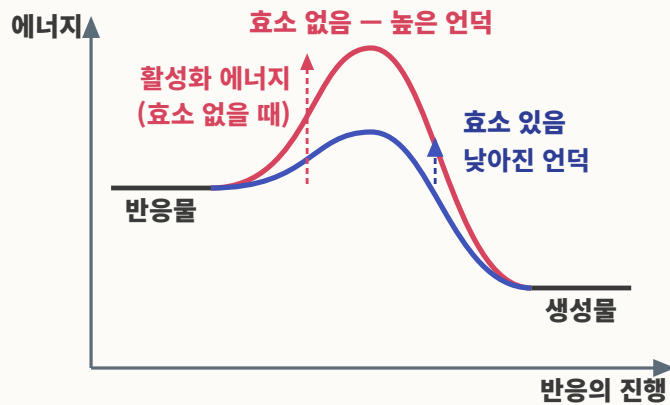
그림 3 | 효소의 작동 원리 — 활성화 에너지 언덕을 낮추고, 짝이 맞는 기질만 골라 뚫고, 반응 후에도 남는다
