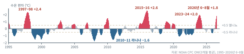
그림 5 | 동태평양 수온 편차 실측 - 빨강 엘니뇨, 파랑 라니냐. 2026년 9월 NOAA 엘니뇨 주의보
