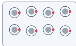
부도체 (유리·고무) 전자가 원자에 붙들림 → 안 통한다
