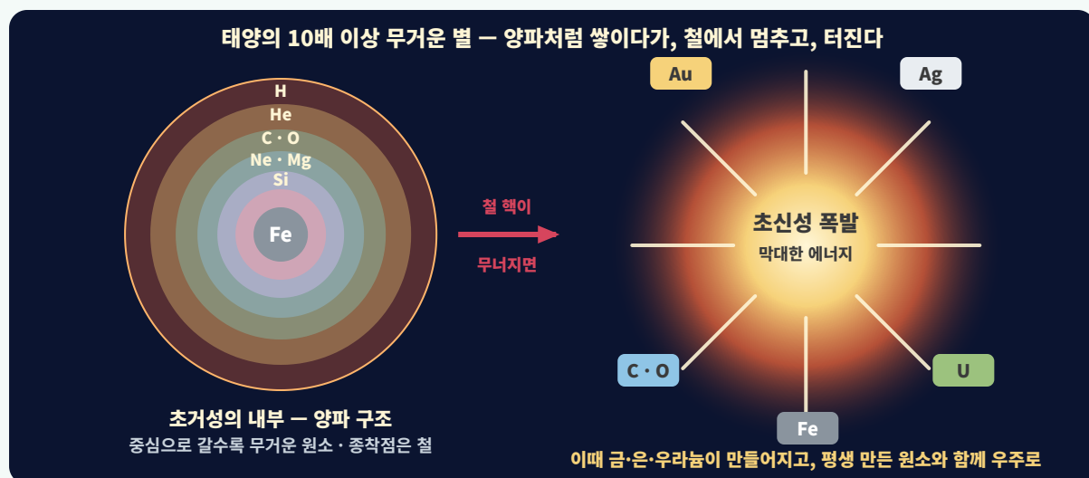
그림 3 | 무거운 별의 최후 — 층층이 원소를 쌓다가 철에서 멈추고, 초신성 폭발로 철보다 무거운 원소까지 만들어 내보낸다
