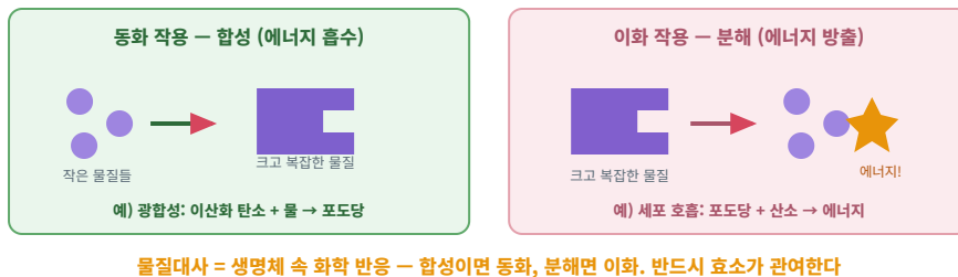
그림 2 | 동화 작용과 이화 작용 — 만들 때는 에너지를 넣고, 부술 때는 에너지가 나온다
