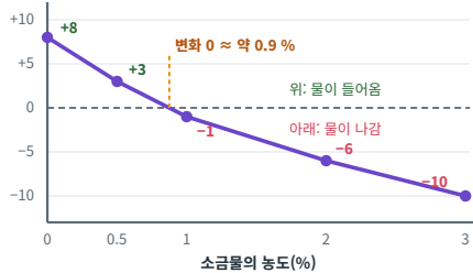
감자 막대의 질량 변화율(%)
