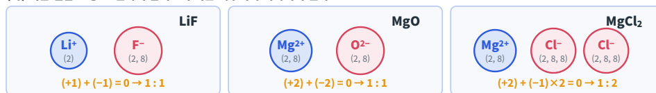
그림 5 | (가) 이온 결합의 형성 — 전자가 이동하고 반대 전하의 이온이 끌어당긴다 (나) 이온 결합 물질의 화학식
