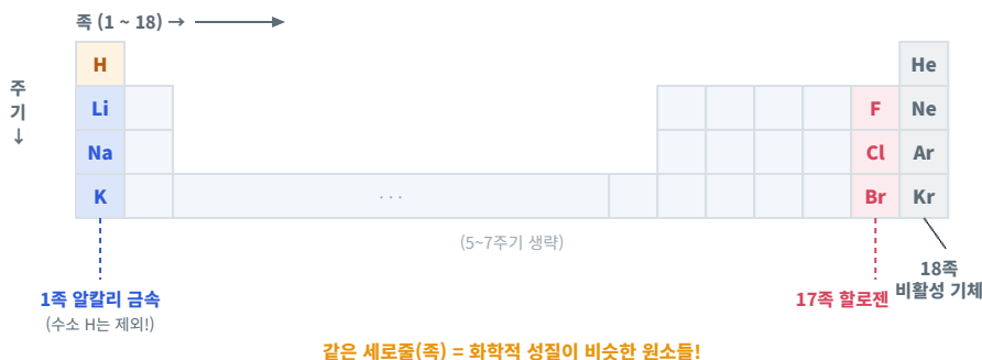
그림 1 | 주기율표의 구조 — 세로줄이 족, 가로줄이 주기. 같은 족 원소는 성질이 닮았다
