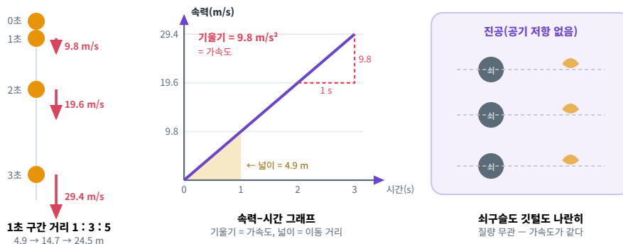
그림 2 | 자유 낙하 — 가속도 약 9.8 \text{ m/s}^2 (매초 9.8 m/s씩), 공기 저항이 없으면 질량과 무관하게 함께 떨어진다
