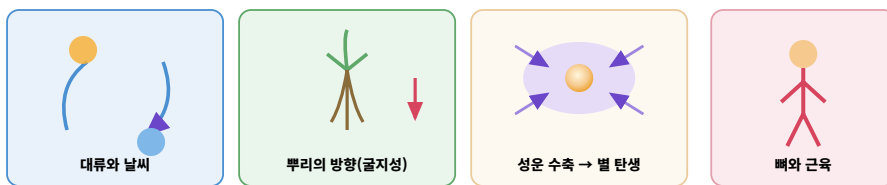
사과를 떨어뜨리는 힘 = 별을 빛는 힘 — 중력은 지구시스템의 조용한 설계자
