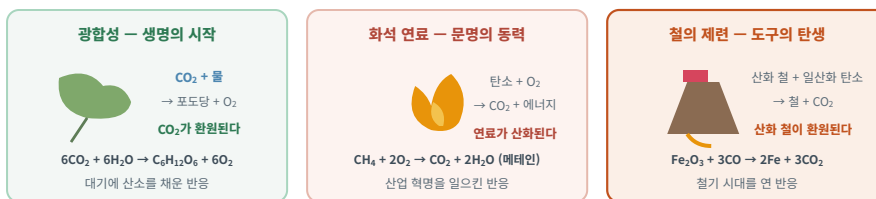
역사를 바꾼 세 반응 — 공통점은 '산소의 이동'
