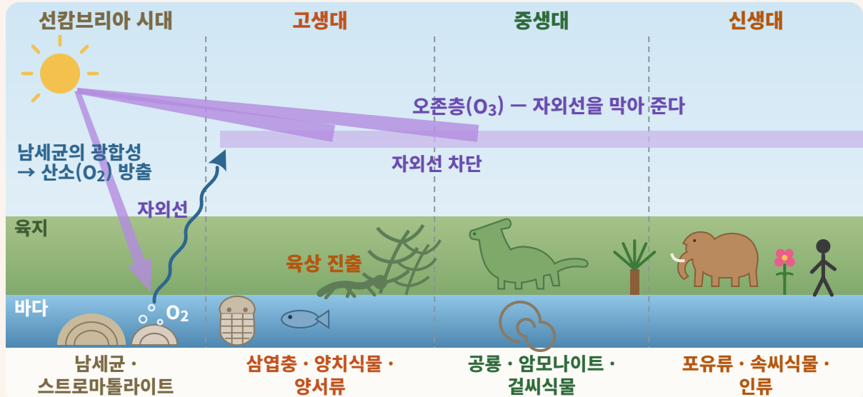
그림 3 | 지질시대의 생물 — 남세균의 산소가 오존층을 만들고, 오존층이 자외선을 막자 생물이 육지로 올라왔다
