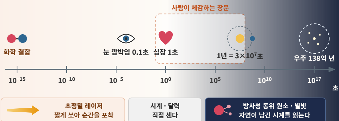
그림 3 | 시간 규모의 사다리 — 화학 반응의 찰나( 10^{-15} 초)에서 우주의 나이(138억 년)까지, 그리고 각 규모를 재는 방법
