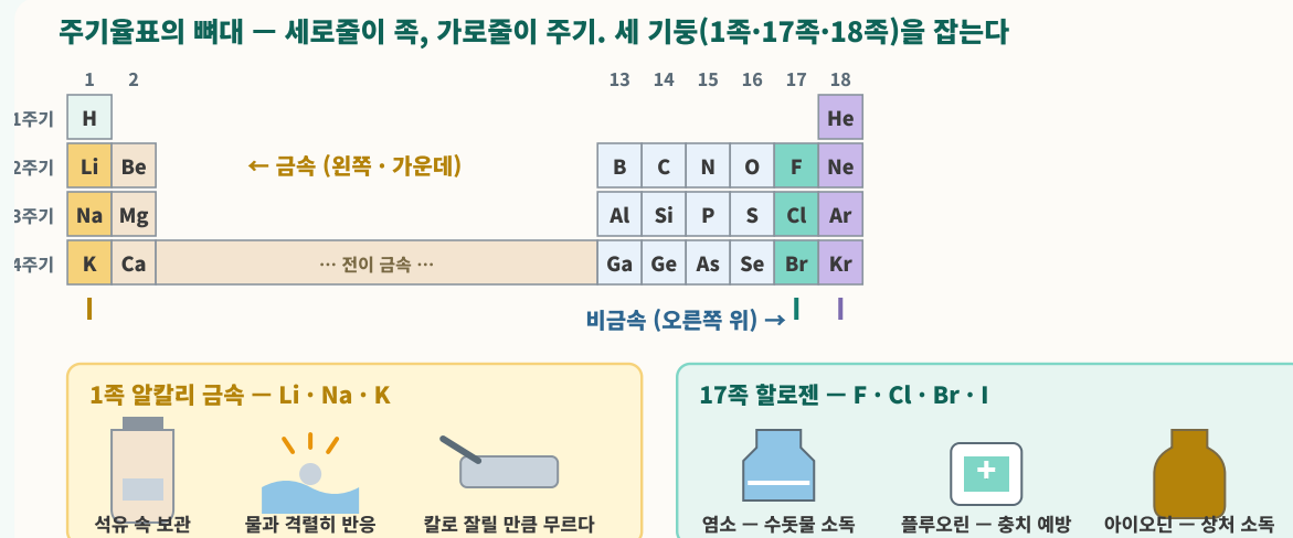
그림 1 | 주기율표의 구조와 두 가족 — 같은 족 원소는 행동이 닮았다. 수소(H)는 1족이지만 알칼리 금속이 아니다
