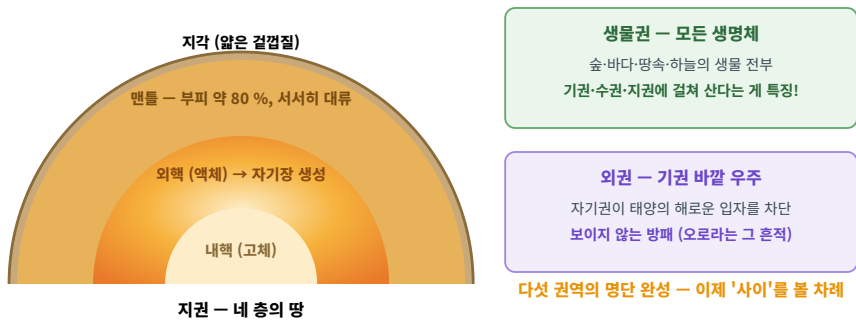
그림 4 | 지권의 층상 구조와 생물권·외권 — 외핵의 흐름이 만든 자기장이 외권에서 방패가 된다
