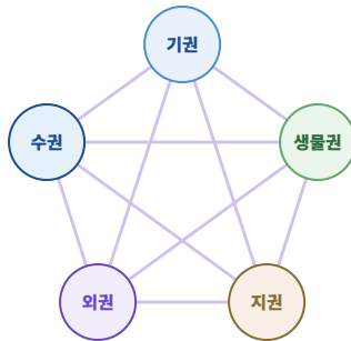
다섯 권역 사이의 연결망이다
