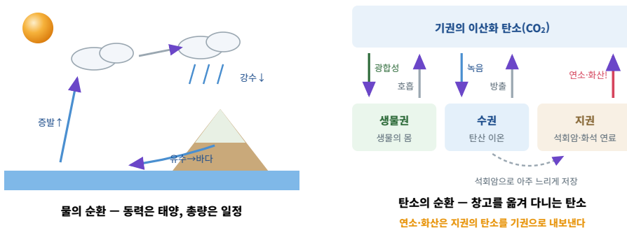
그림 7 | 물과 탄소의 순환 — 물질은 권역 사이를 돌고, 그 동력은 태양 에너지다
