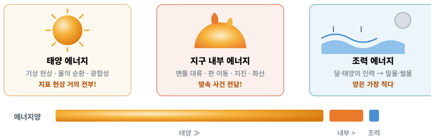
그림 5 | 세 에너지원의 담당 구역과 크기 — 태양 >> 지구 내부 > 조력
