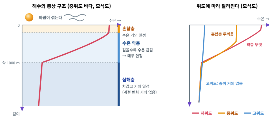
그림 3 | 해수의 층상 구조 — 바람이 섞는 혼합층, 안정한 수온 약층, 차갑고 일정한 심해층
