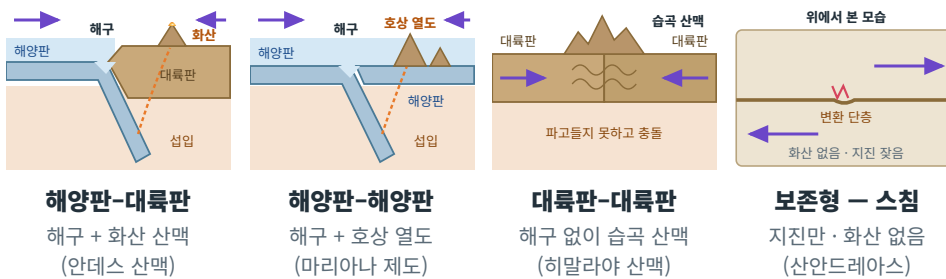
그림 3 | 수렴형 경계 세 가지와 보존형 경계 — 무거운 판은 가라앉고, 대륙판끼리는 솟고, 스치면 흔들린다
