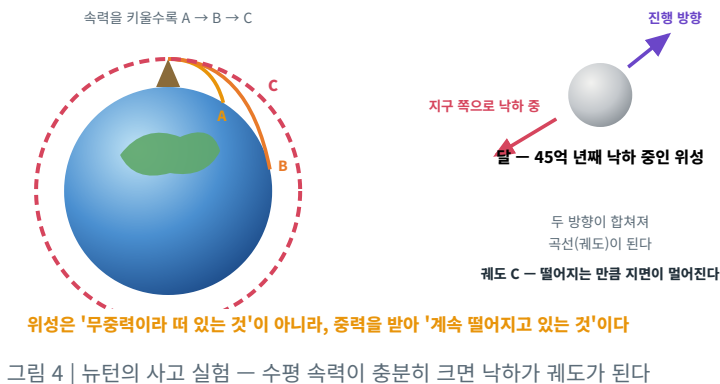
그림 4 | 뉴턴의 사고 실험 — 수평 속력이 충분히 크면 낙하가 궤도가 된다
