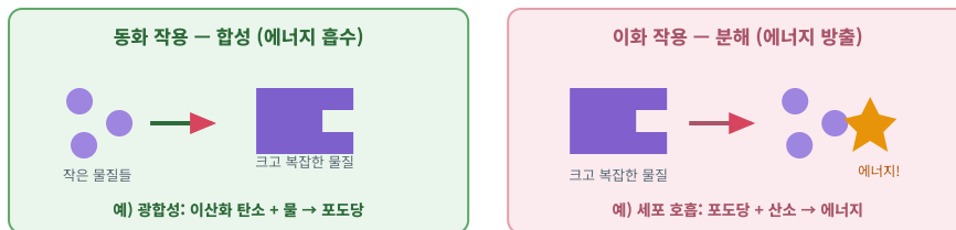
그림 2 | 동화 작용과 이화 작용 — 만들 때는 에너지를 넣고, 부술 때는 에너지가 나온다
