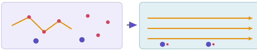
원자 생성 전 : 불투명한 우주 빛이 자유 전자에 사라되어 지지 못함
