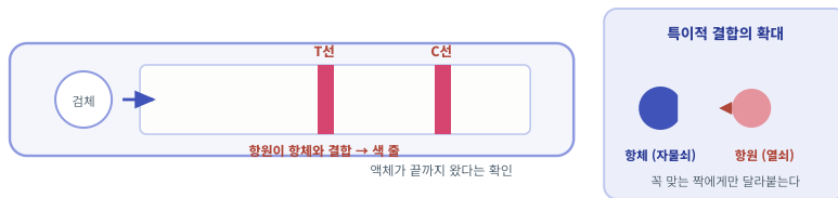
신속 항원 검사 키트 — 자물쇠(항체)와 열쇠(항원)
