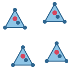
감람석 사면체가 따로따로
