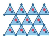
흑운모 얇게 잘 벗겨진다
