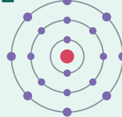
그림 3 | 비활성 기체의 전자 배치와 결합의 이유 — 모든 화학 결합은 이 '가득 찬 바깥 껍질'을 향한다
