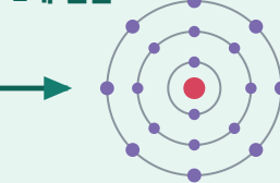
그림 3 | 비활성 기체의 전자 배치와 결합의 이유 — 모든 화학 결합은 이 '가득 찬 바깥 껍질'을 향한다
