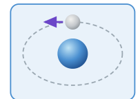
(다) 지구 둘레를 도는 달
