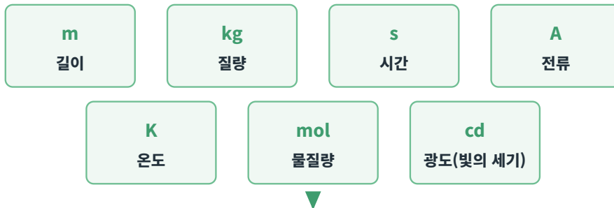
국제단위계(SI)의 기본량 7가지 — 자연을 쓰는 알파벳
