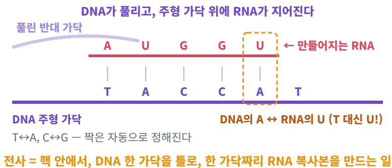
그림 3 | 전사 — 주형 가닥 TAC...에서 RNA AUG...가 태어난다
