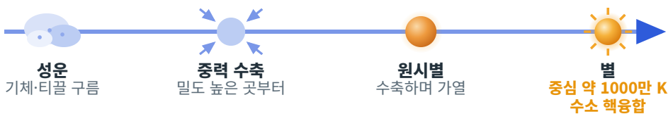
그림 1 | 별의 탄생 과정 — 성운이 중력으로 수축하고, 중심 온도가 약 1000만 K에 이르러 수소 핵융합이 시작되면 별이 된다
