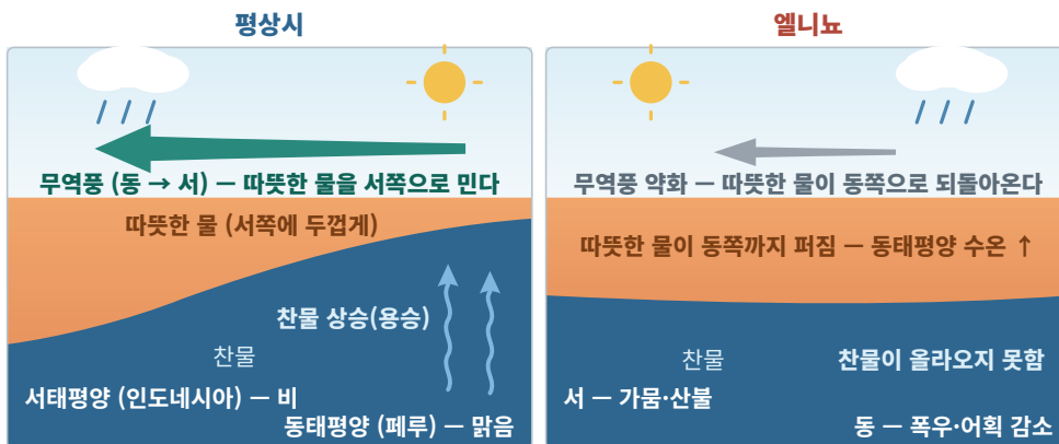
적도 태평양을 옆에서 자른 단면 — 왼쪽이 서쪽, 오른쪽이 동쪽. 주황: 따뜻한 물, 파랑: 찬물
