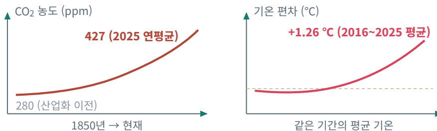
두 개의 상승 곡선 — 원인과 결과
