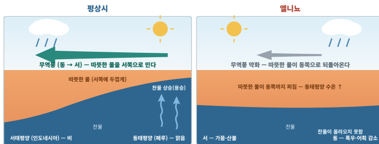
적도 태평양을 옆에서 본 단면 — 왼쪽이 서쪽, 오른쪽이 동쪽. 주황: 따뜻한 물, 파랑: 찬물
