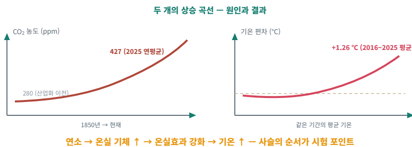
그림 2 | 이산화 탄소 농도와 지구 평균 기온 — 나란히 오르는 두 곡선(개념도 · 수치: NOAA 2025, IGCC 2026)
