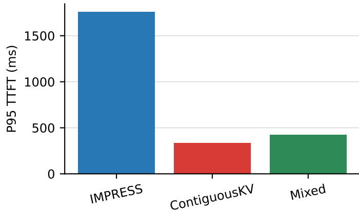
RTE
