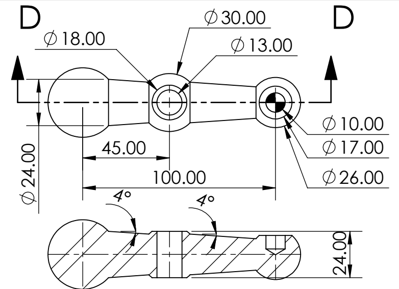
SECTION D-D
