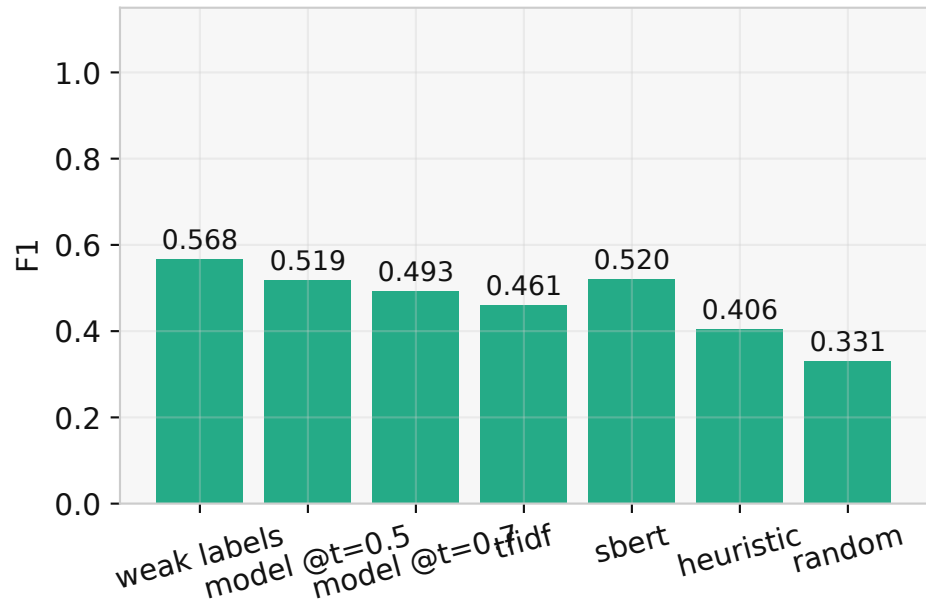
F1
