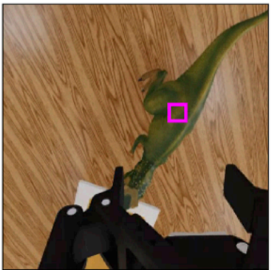
V-JEPA 2
