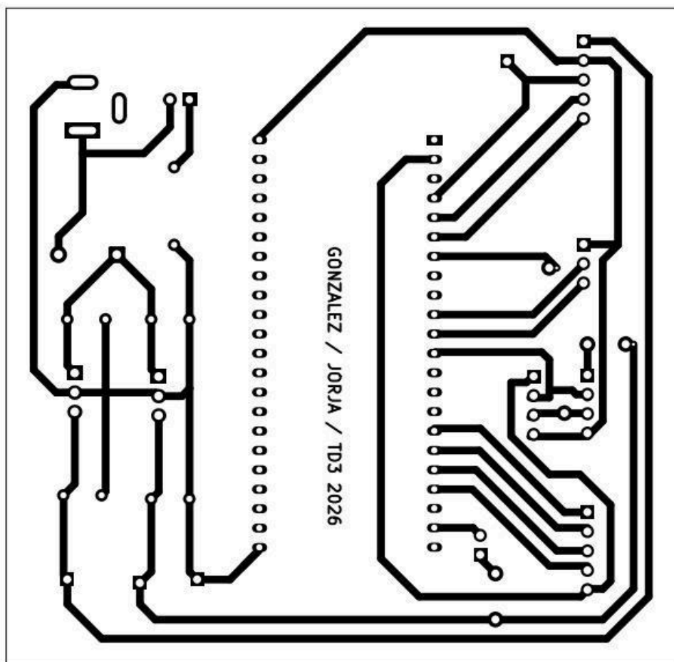
Fig. A3. Diseño del PCB del prototipo.
