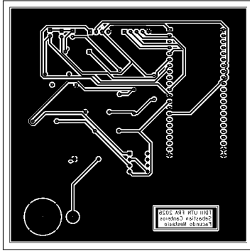
Fig. 9. PCB
