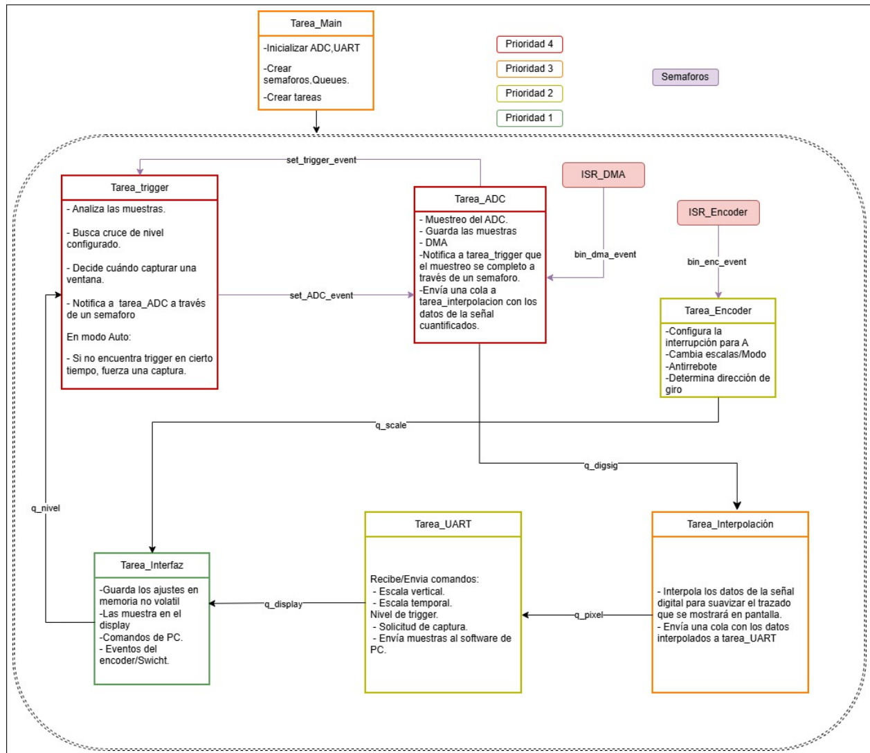
Fig. 7. Diagrama de tareas del osciloscopio.
