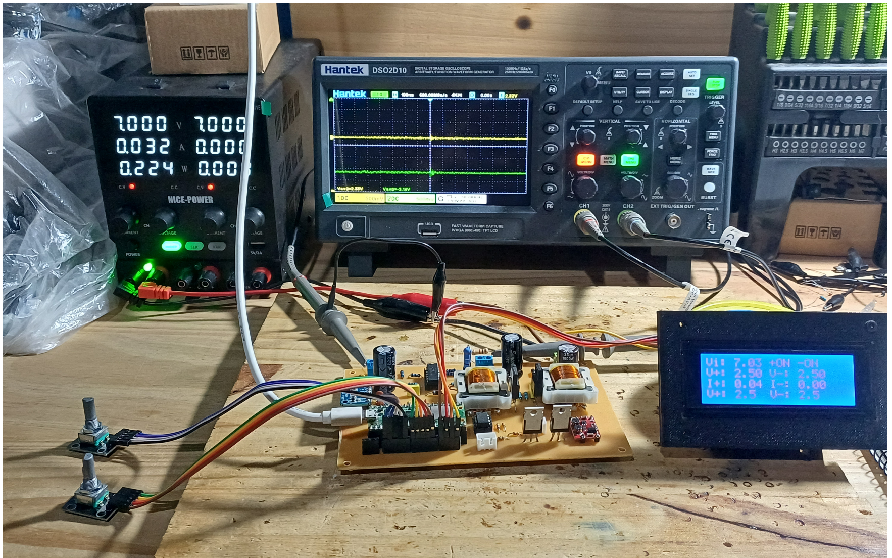
Figura 7. Prototipo completo durante una medición previa a la calibración definitiva. Se observan las dos cargas, los encoders, el LCD, la fuente de laboratorio y los dos canales del osciloscopio Hantek DSO2D10. La diferencia entre instrumental y display motivó las tablas independientes de V_{in} , V_{out} positiva y V_{out} negativa.
