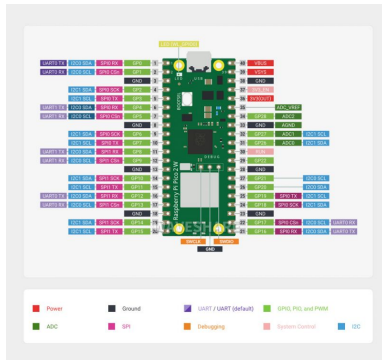
Figura 1. Raspberry Pi Pico 2W y distribución de pines empleada como referencia para la asignación de señales.
