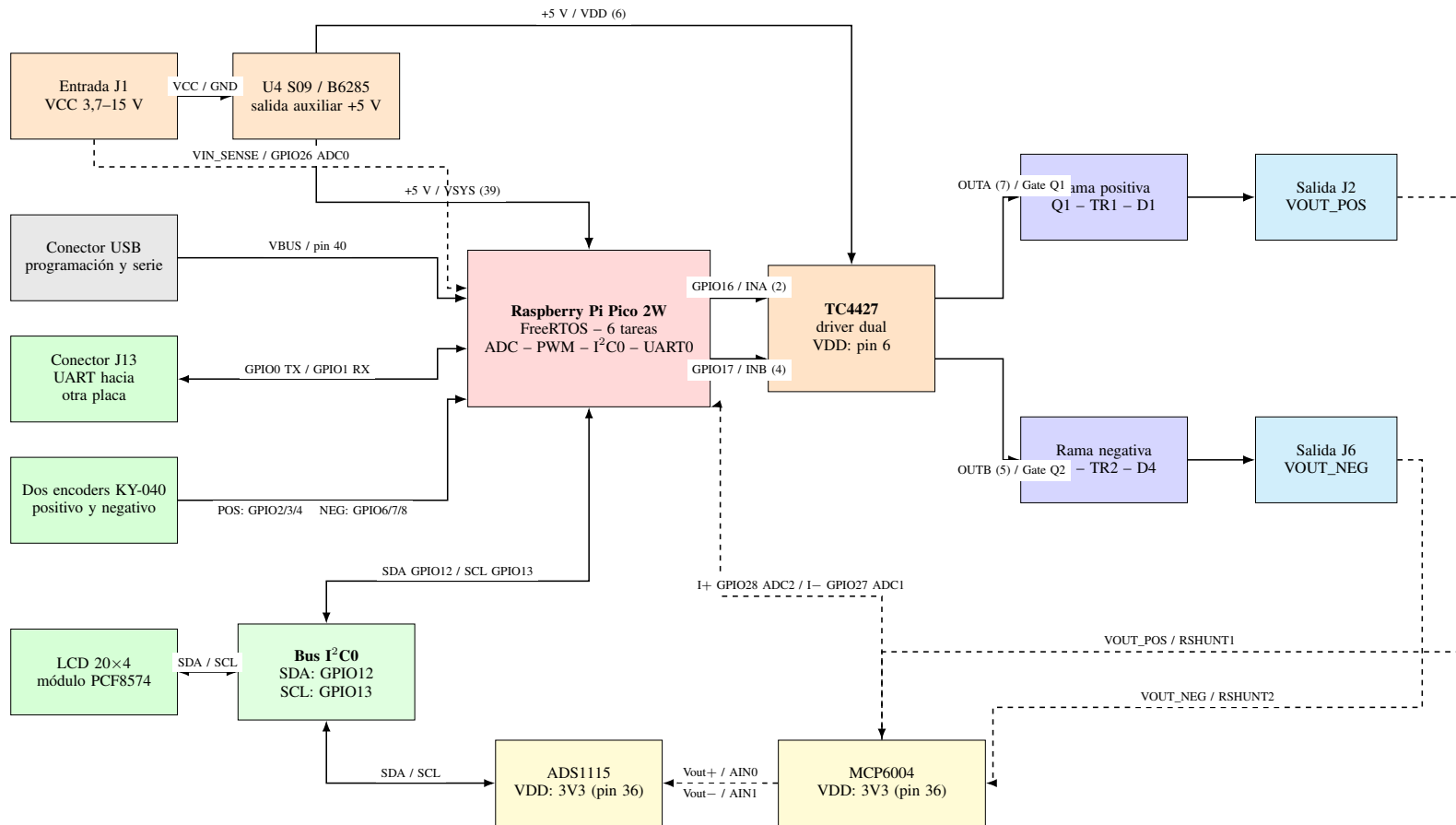
Figura 6. Conexión de los módulos y pines utilizados. Las líneas continuas representan alimentación o señales digitales; las discontinuas corresponden a mediciones analógicas.
