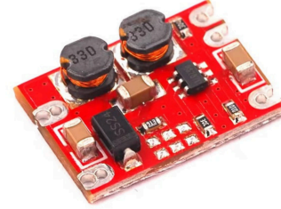
Figura 2. Fotografía real del módulo S09 utilizado para obtener el riel auxiliar de 5 V [9].
