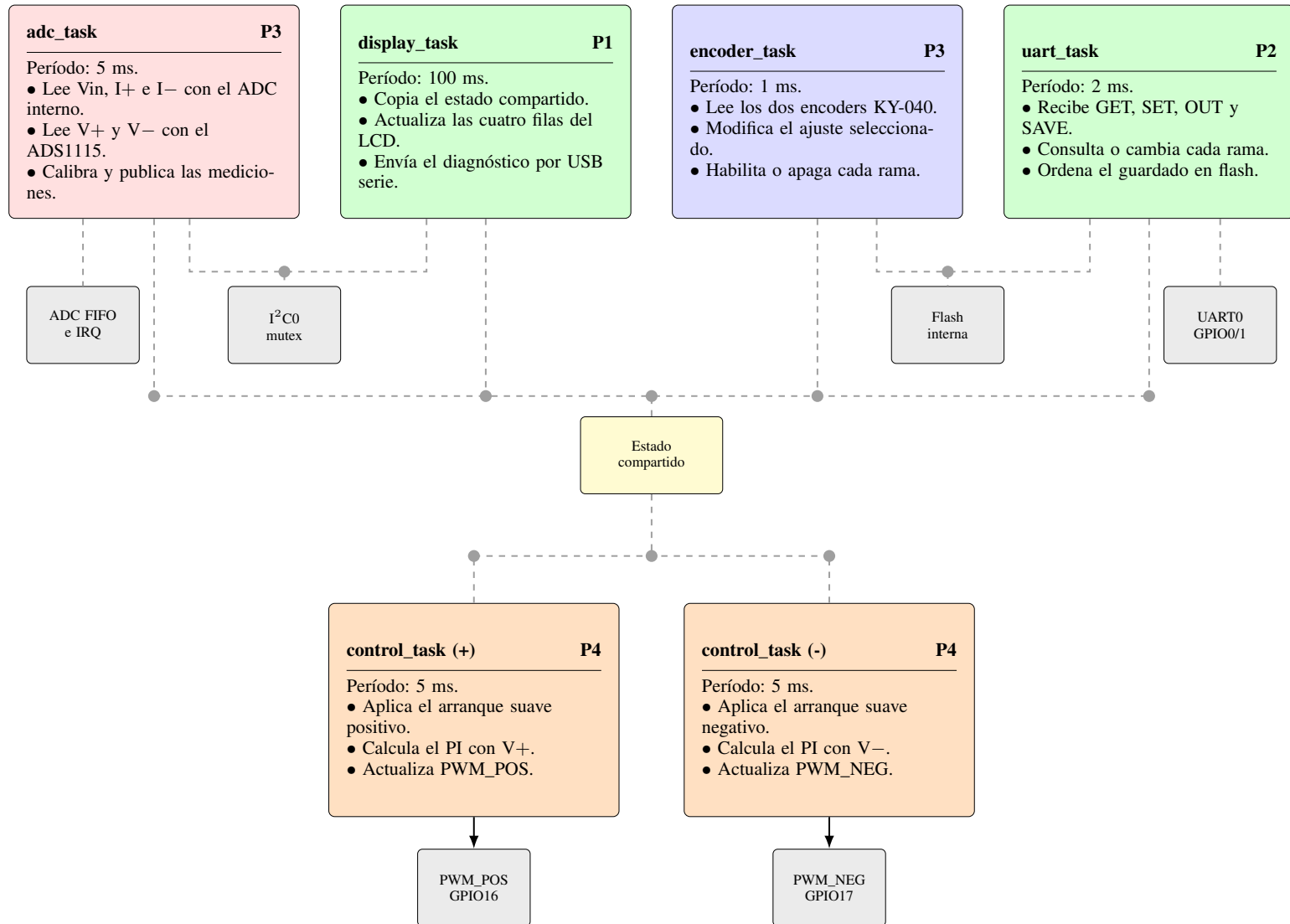
Figura 5. Seis tareas de FreeRTOS y recursos compartidos. La protección rápida se ejecuta en la IRQ del ADC, no como una tarea adicional. Las líneas discontinuas indican acceso a un recurso y las flechas continuas corresponden a las salidas PWM.
