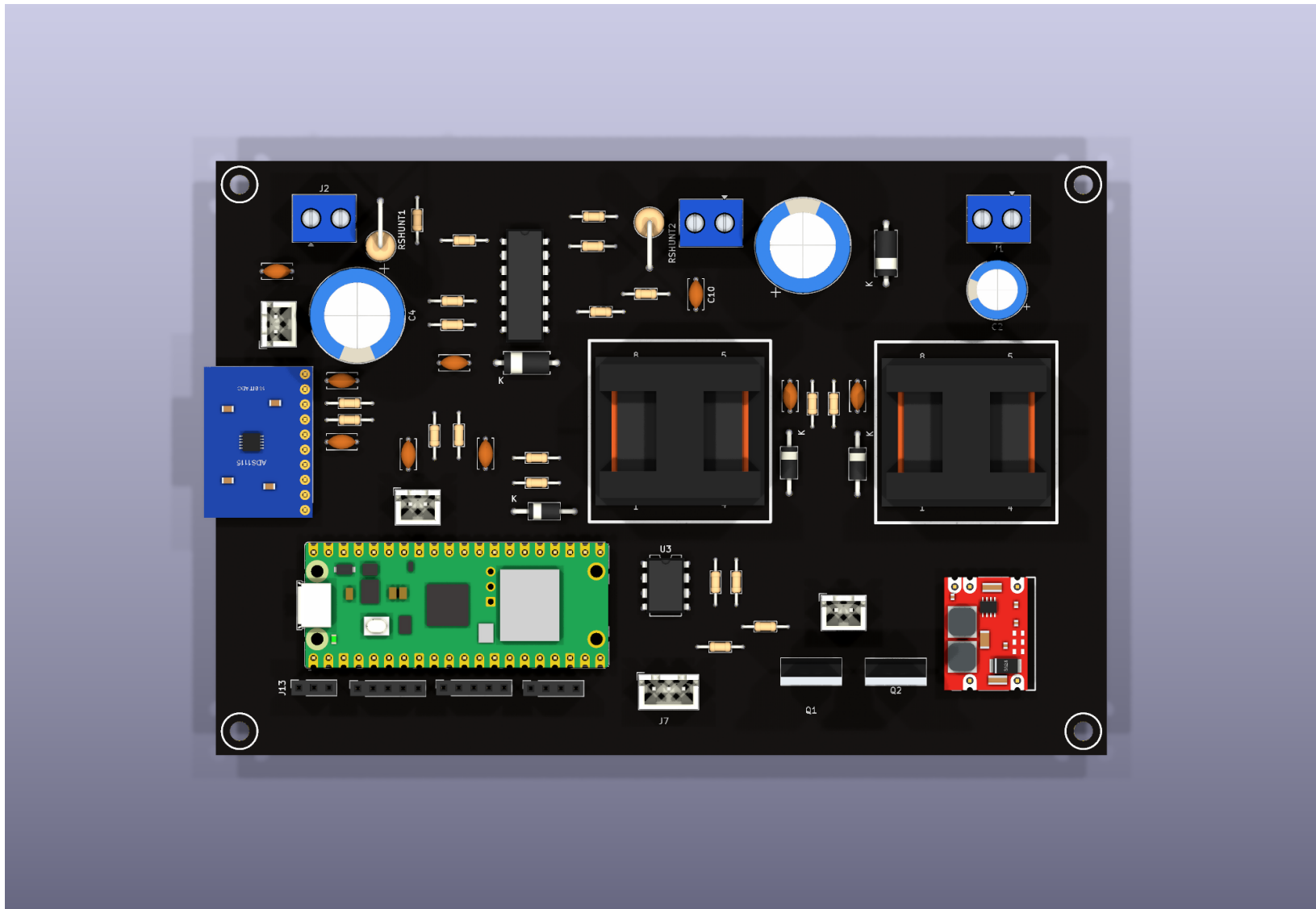
Figura 9. Vista superior completa de la PCB vigente de 150 mm por 100 mm.
