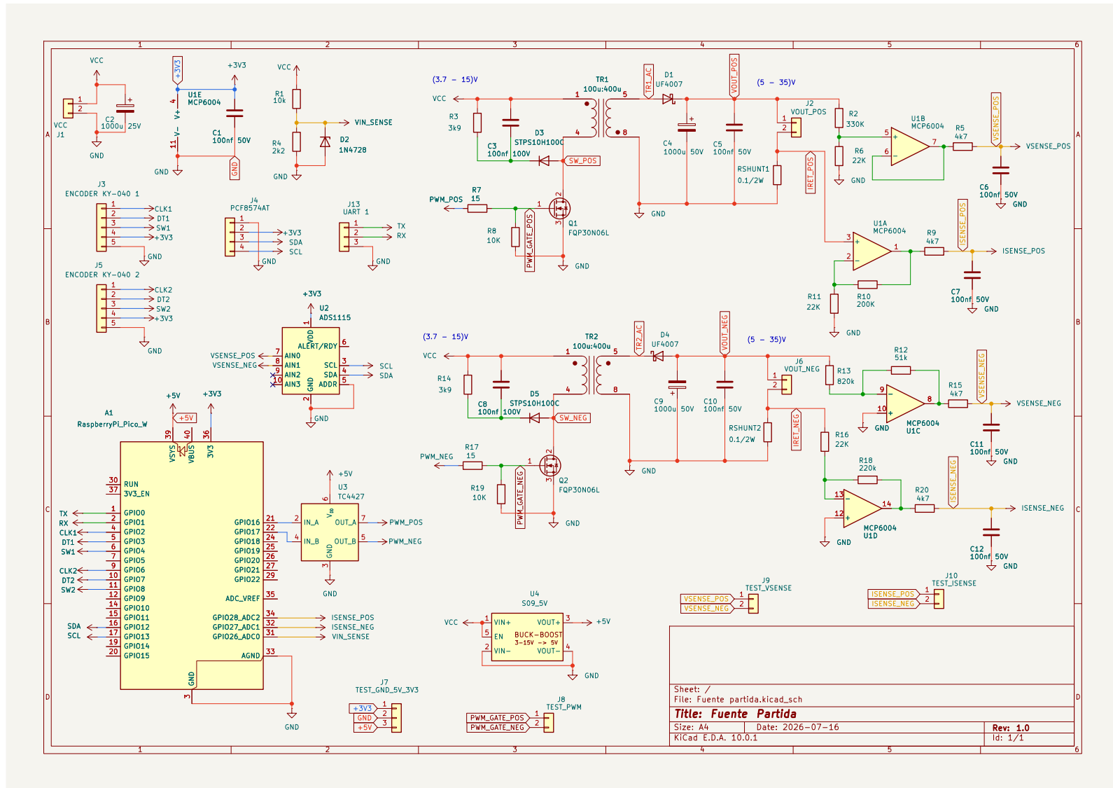
Figura 8. Esquemático completo a color exportado desde el proyecto KiCad vigente.
