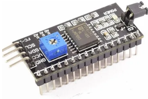
Figura 4. Interfaz PCF8574 empleada por el LCD 20×4.
