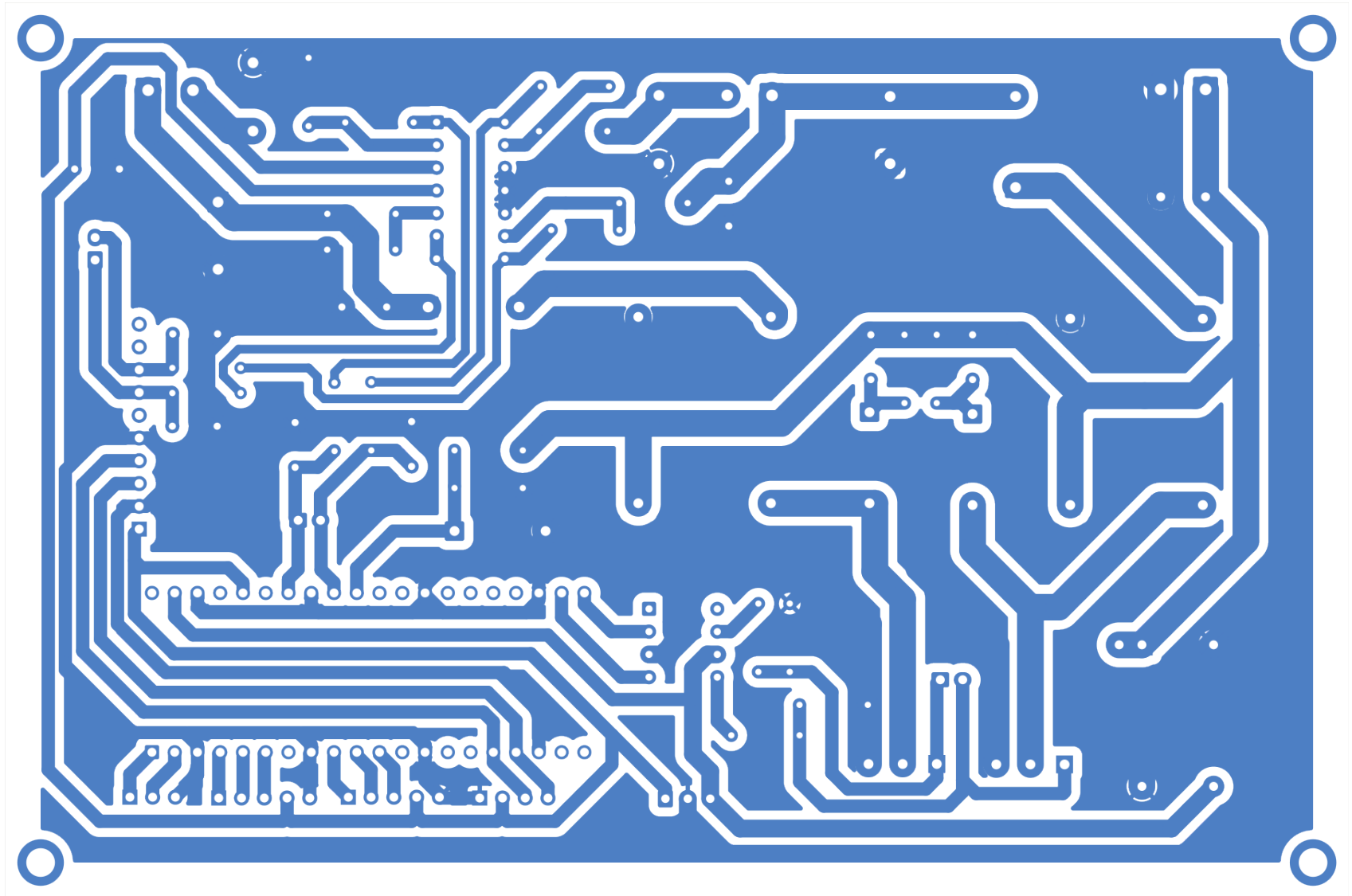
Figura 10. Capa B.Cu vigente exportada desde KiCad, con el ruteo de cobre y los taladros de la PCB.
