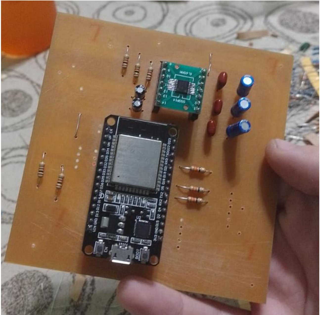
Anexo 4 PCB ensamblado
