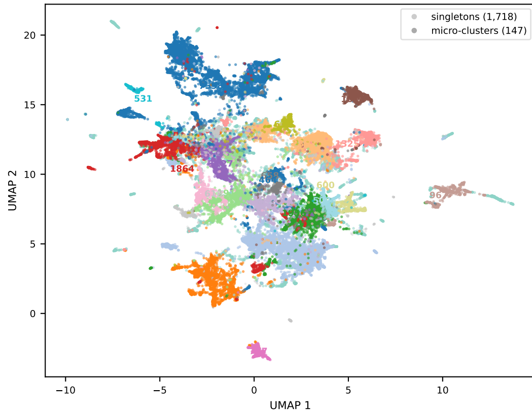
1 · Cluster map
