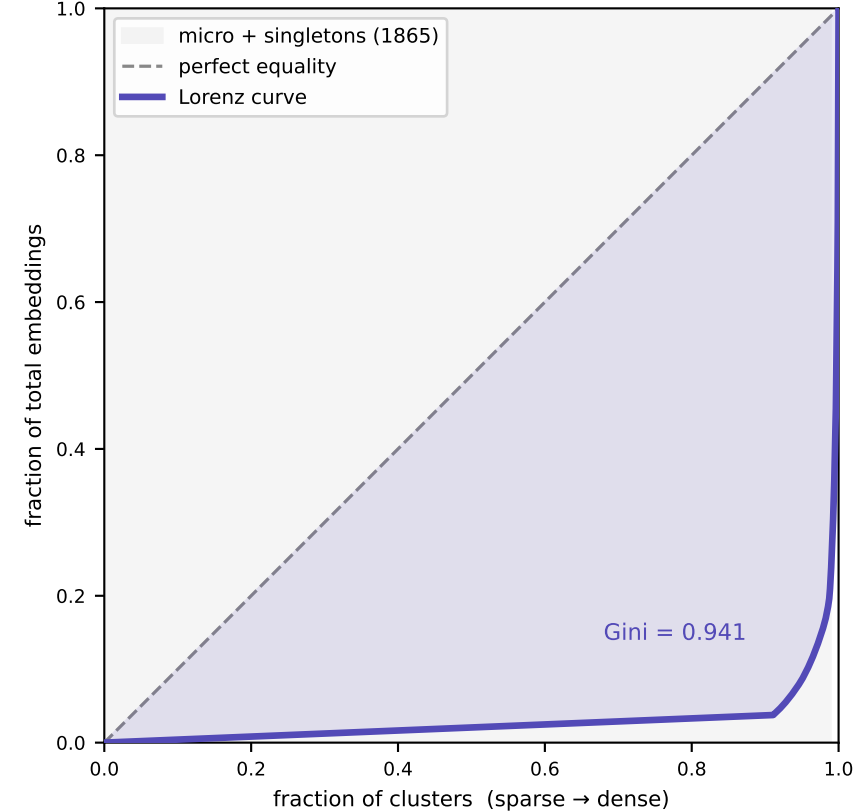
3 · Lorenz curve
