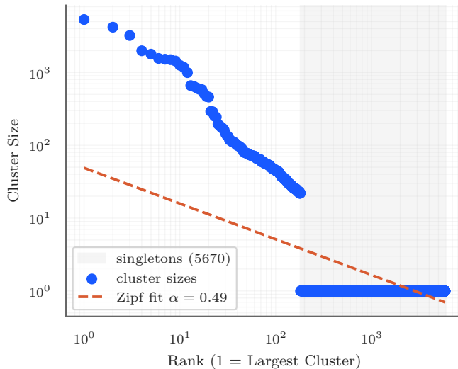
2 · Rank-Size
