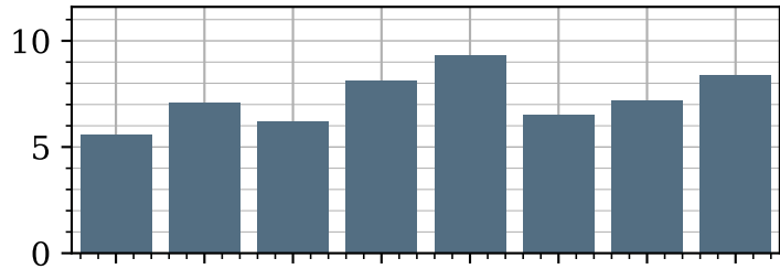
Text8
