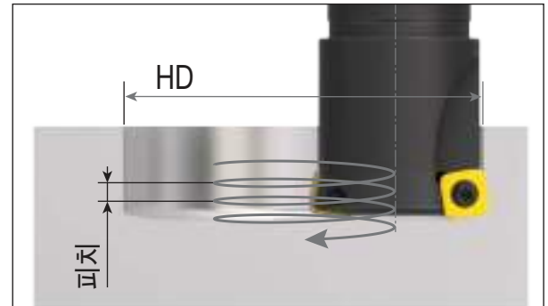
헬리컬 램핑 가공
