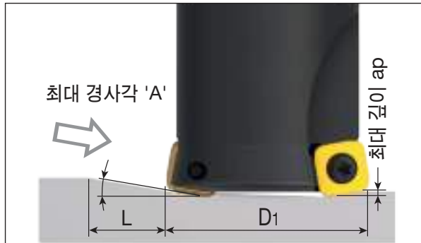
직선 램핑 가공
