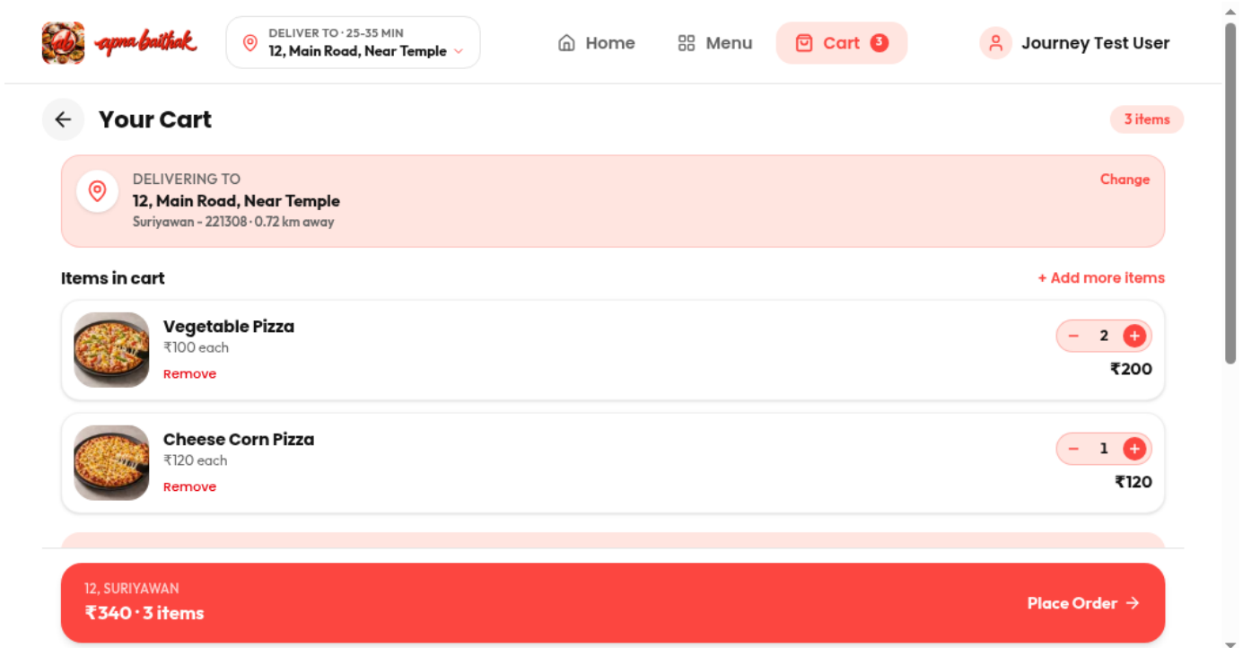
Screenshot: journey-24-cart-view.png
