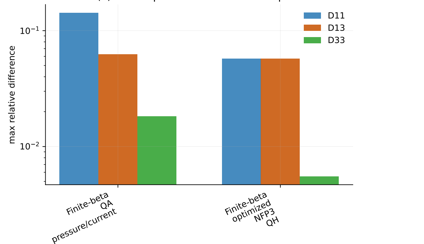
(d) Boozer path vs VMEC-harmonic path
