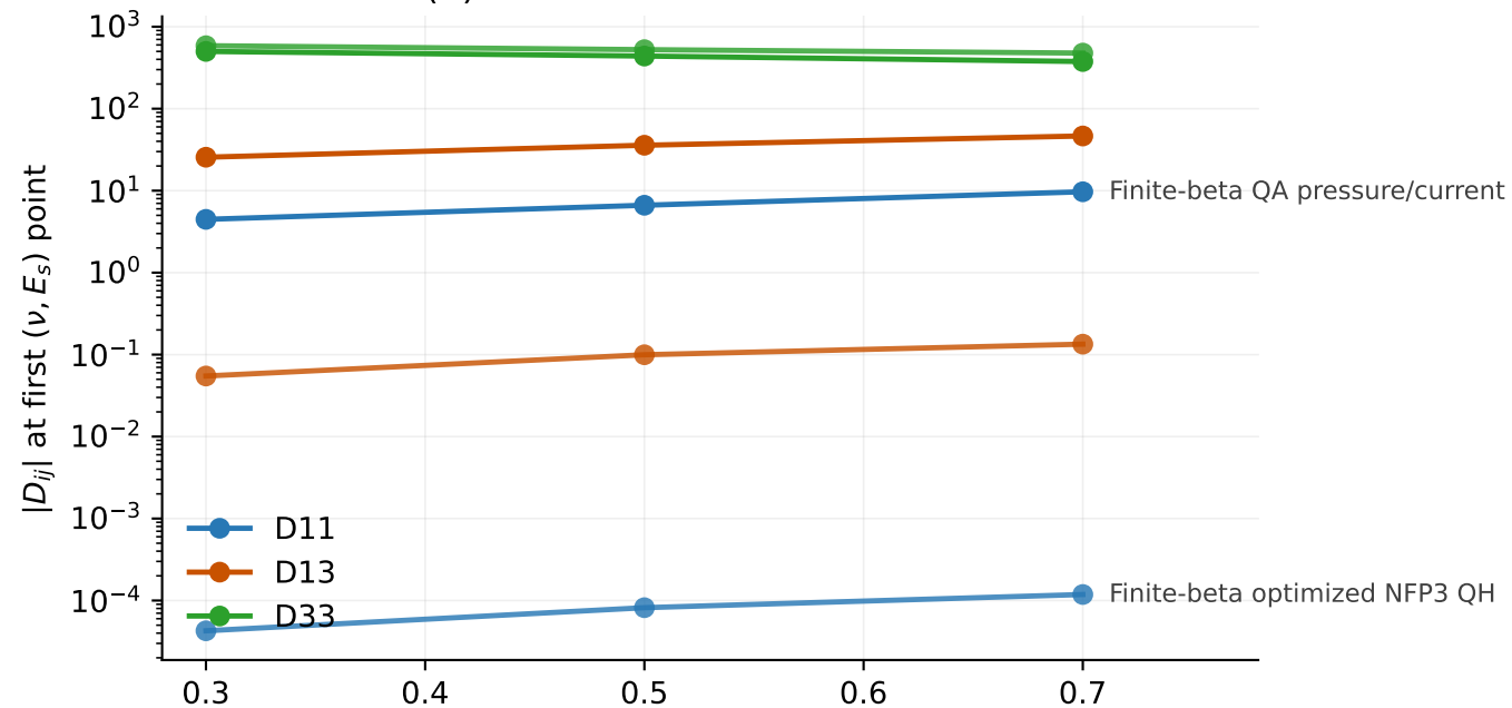
(d) Boozer path vs VMEC-harmonic path
