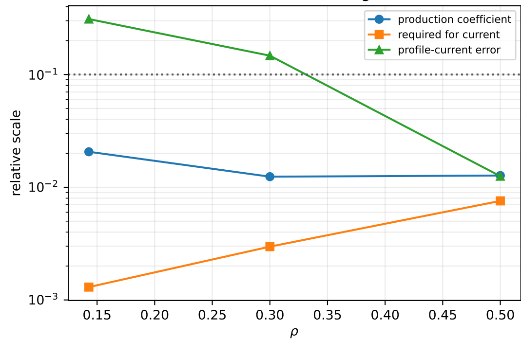
(d) Ladder error budget
