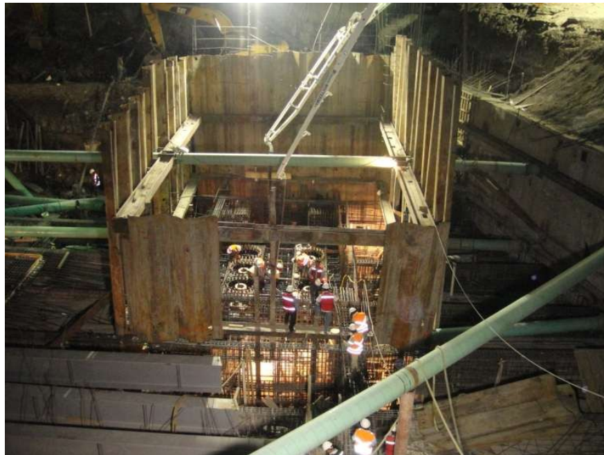
12. Colado de dado de cimentación, mayo de 2011
