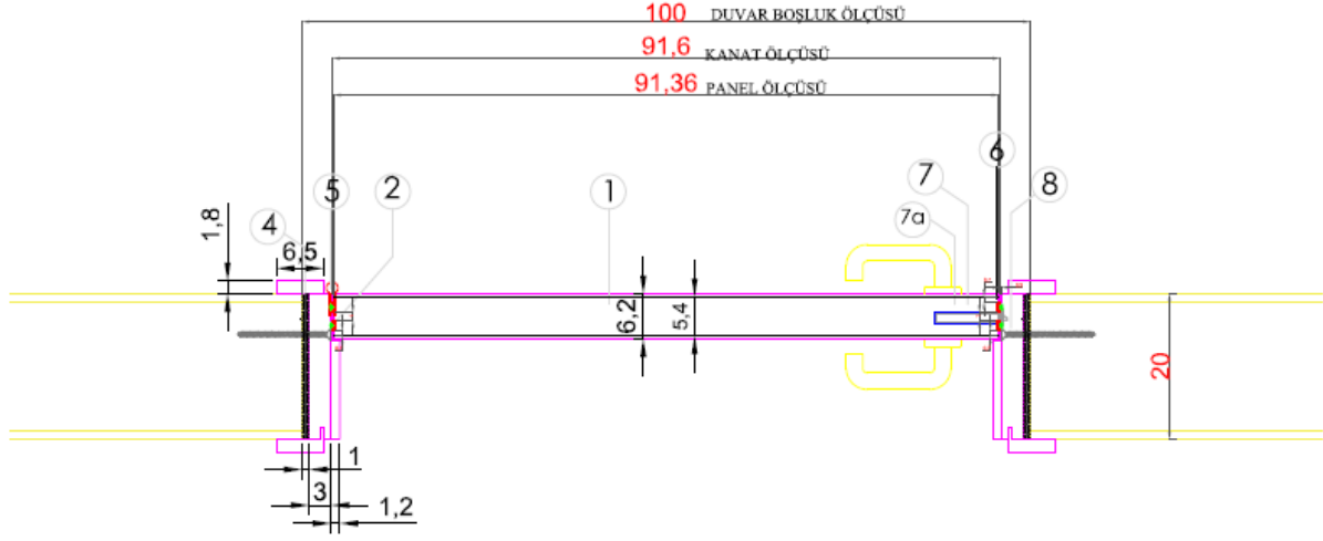
Şekil 7: Kapı No.2'nin enine kesit detayları.
