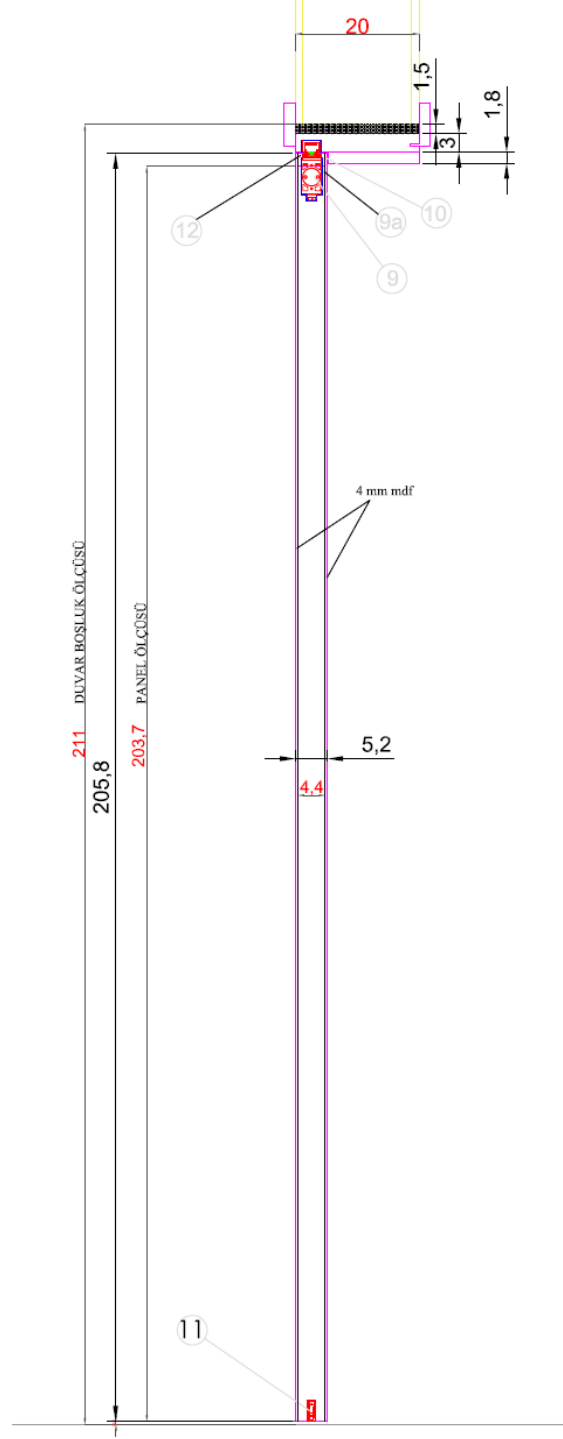
Şekil 2: Kapı No.1'in boyuna kesit detayları.
