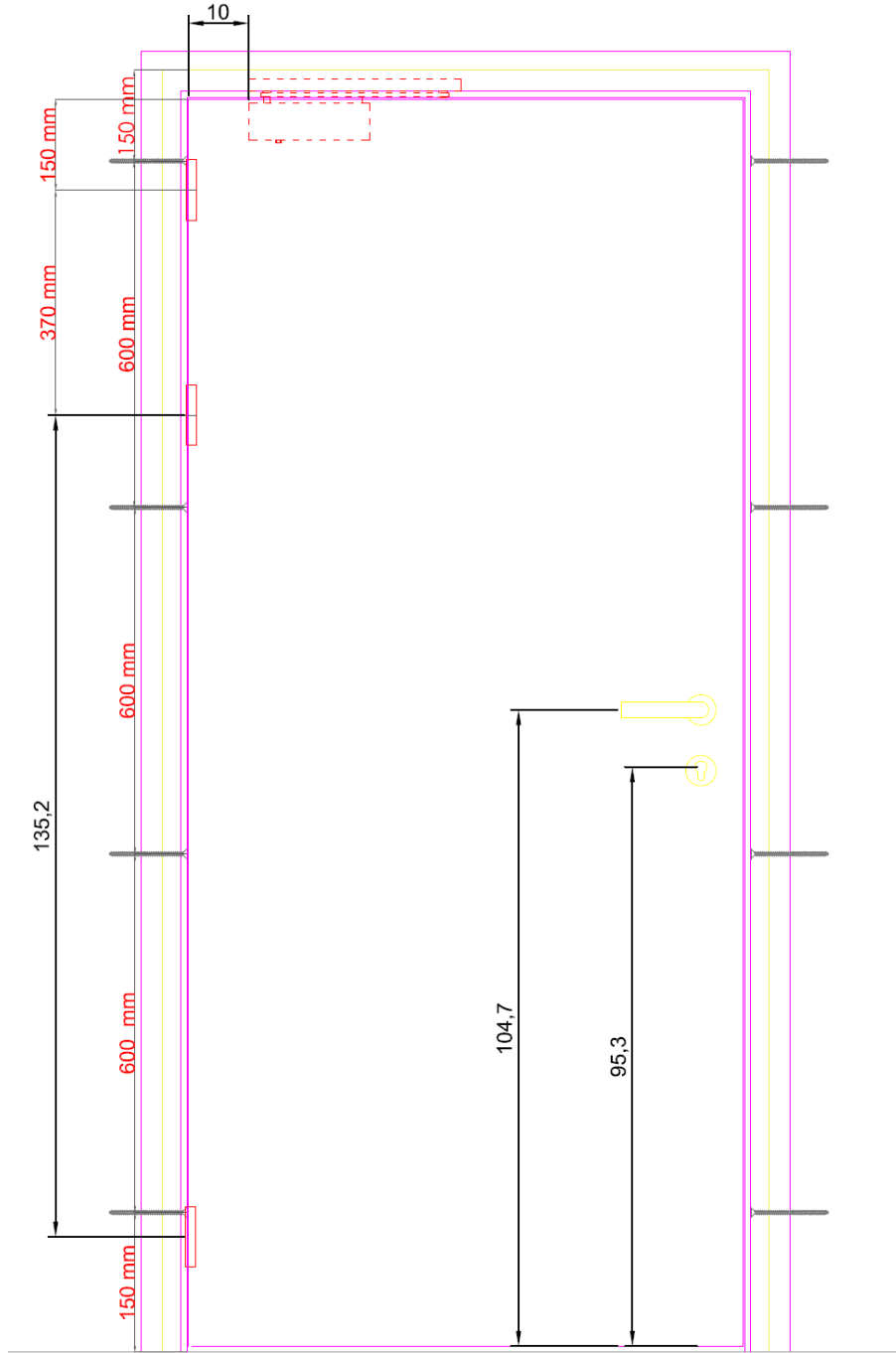
Şekil 1: Kapı No.1'in aleve maruz kalan taraf detayları.
