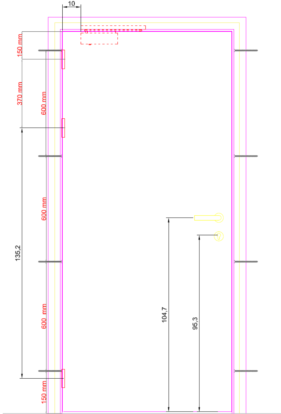
Şekil 5: Kapı No.2'nin aleve maruz kalan taraf detayları.
