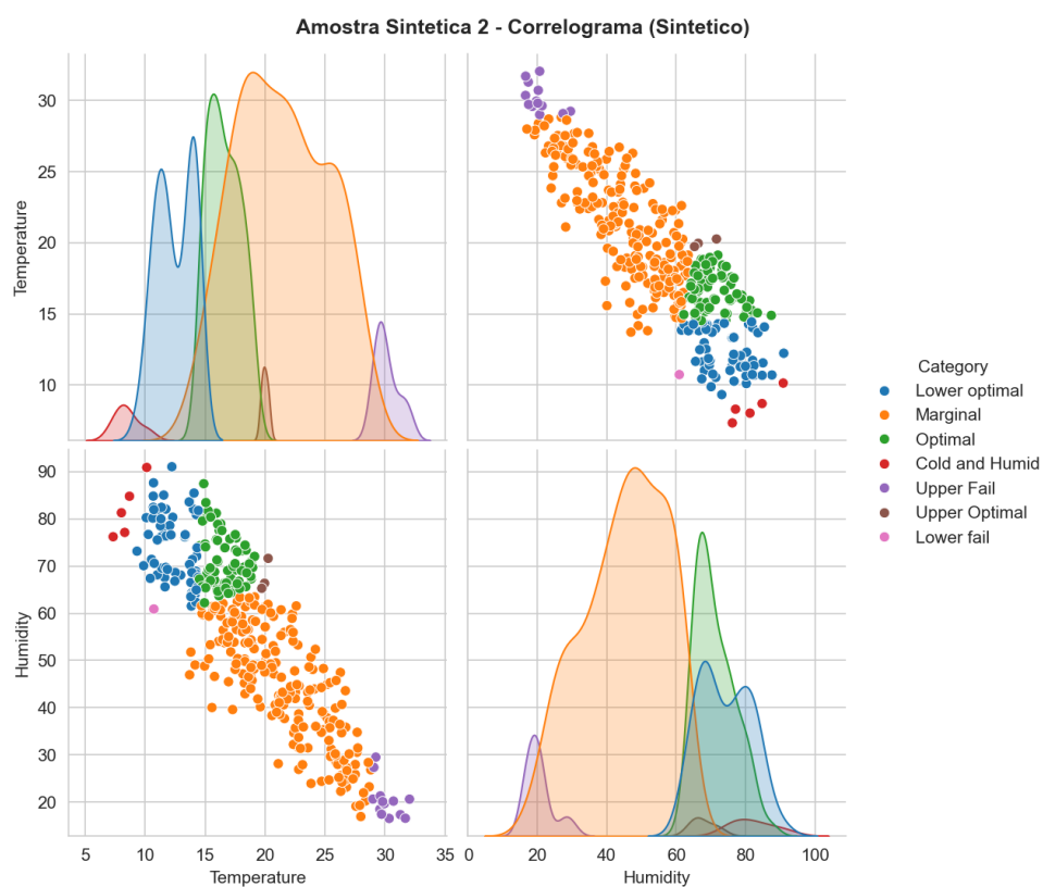
Figura 4 – Correlogramas de Temperatura vs Umidade classificados por kNN (Round 2)
