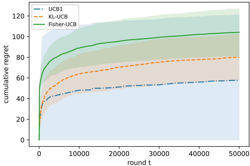
Binomial adverse ( \rho > 0, p > 1/2 )
