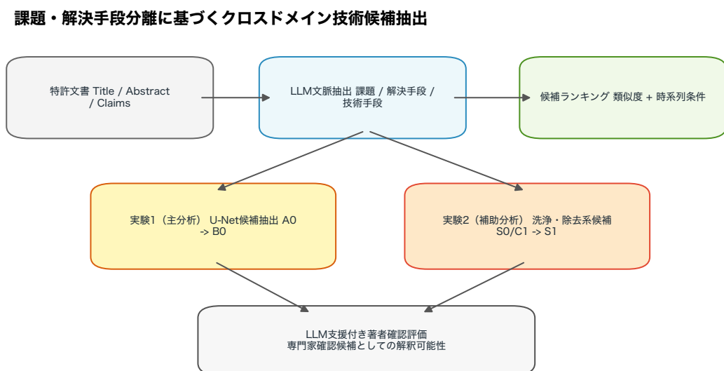
図 1.1: 本研究の全体像。特許文書を課題文脈と解決手段文脈に分離し、専門家確認候補を抽出するスクリーニング手法として整理する。
