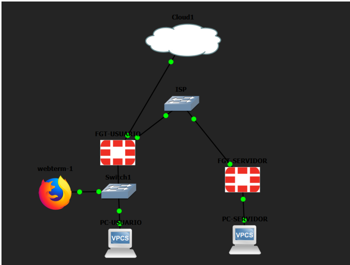
Topología correspondiente a la Infraestructura 1.
