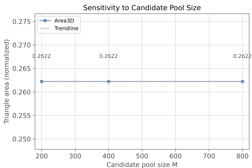
图 9: 候选规模 M 与最优三角形面积的关系（strict 映射）。
