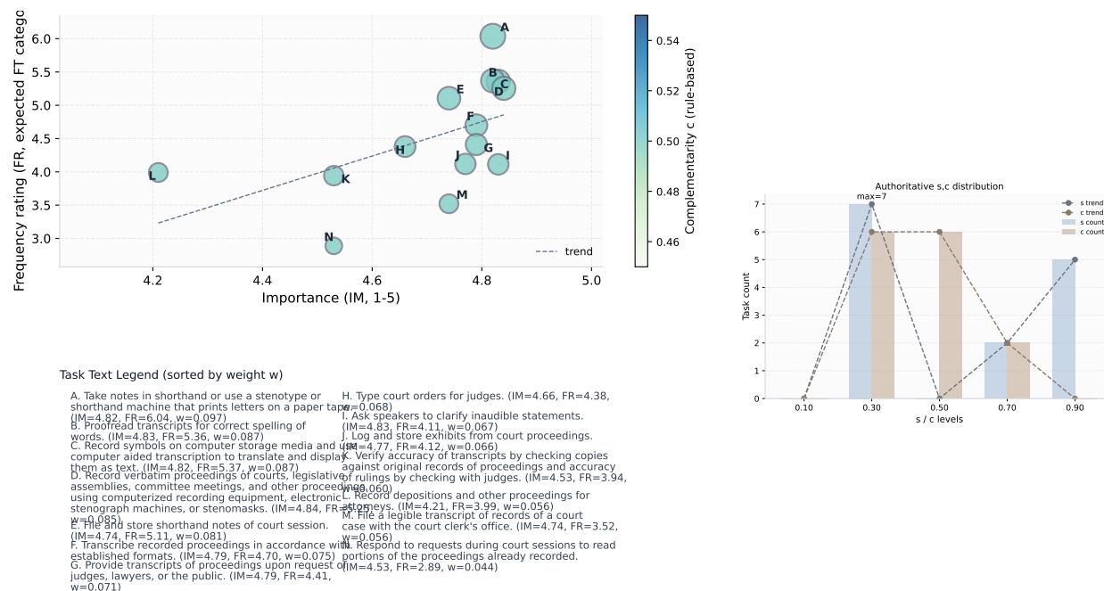
图 10: 职业 27-3092.00 的任务 DNA 与权威 s, c 分布。(a) 任务 DNA 权重分布: IM–FR 散点图, 点面积与 w 成正比; (b) 权威 s, c 档位分布。
